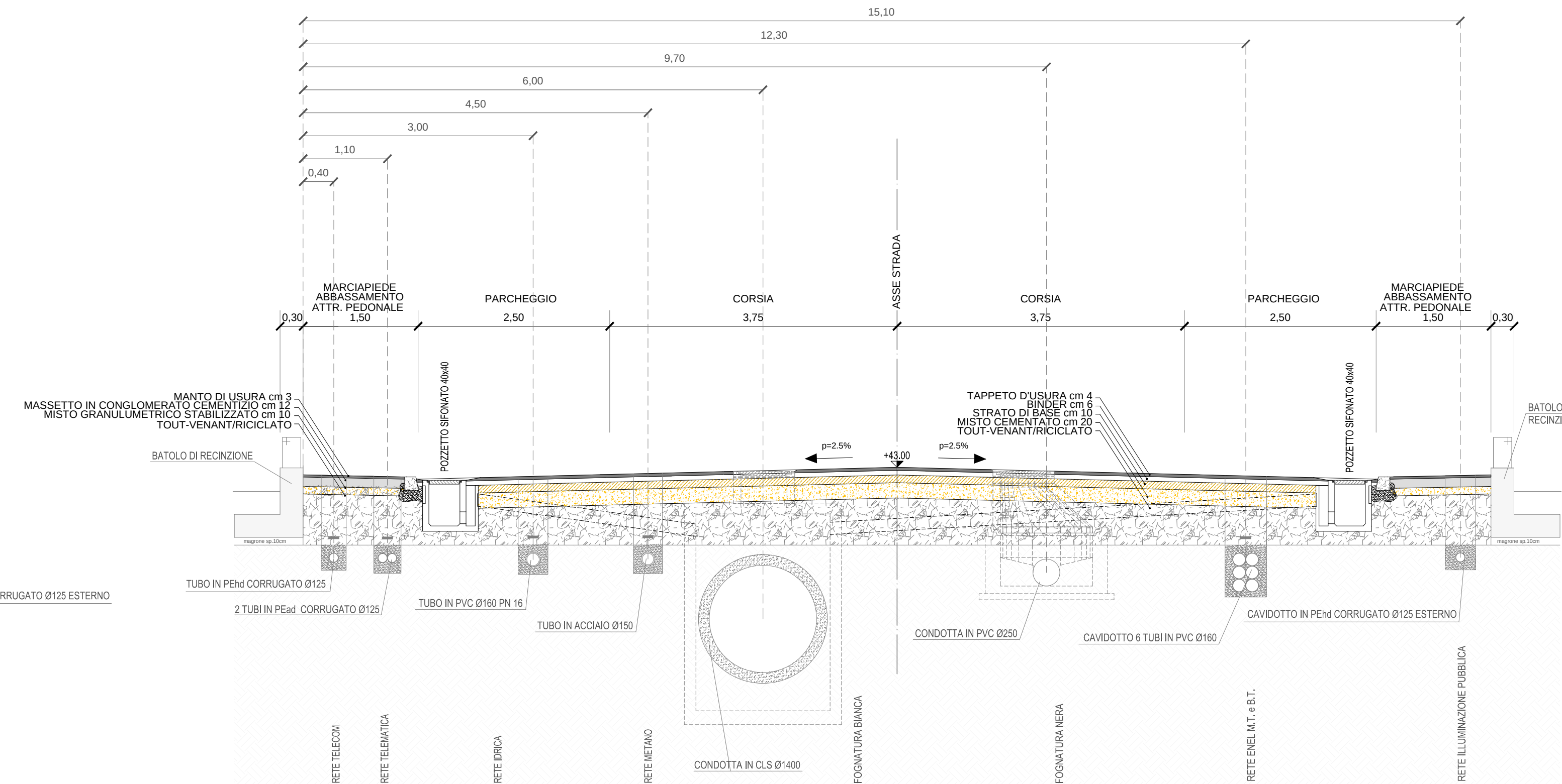
SEZIONE TIPO D-D SCALA 1:50
