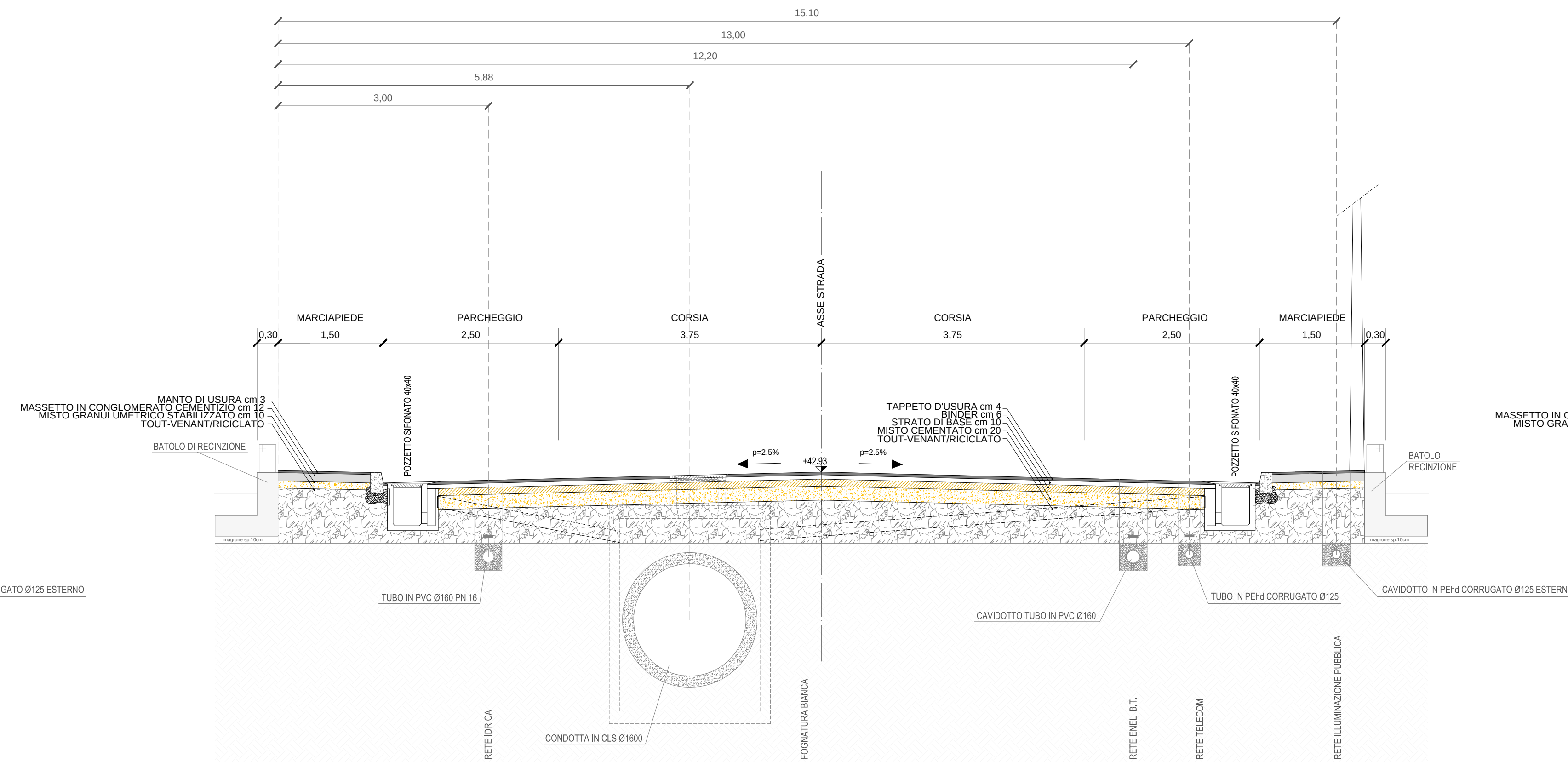
SEZIONE TIPO C-C SCALA 1:50
