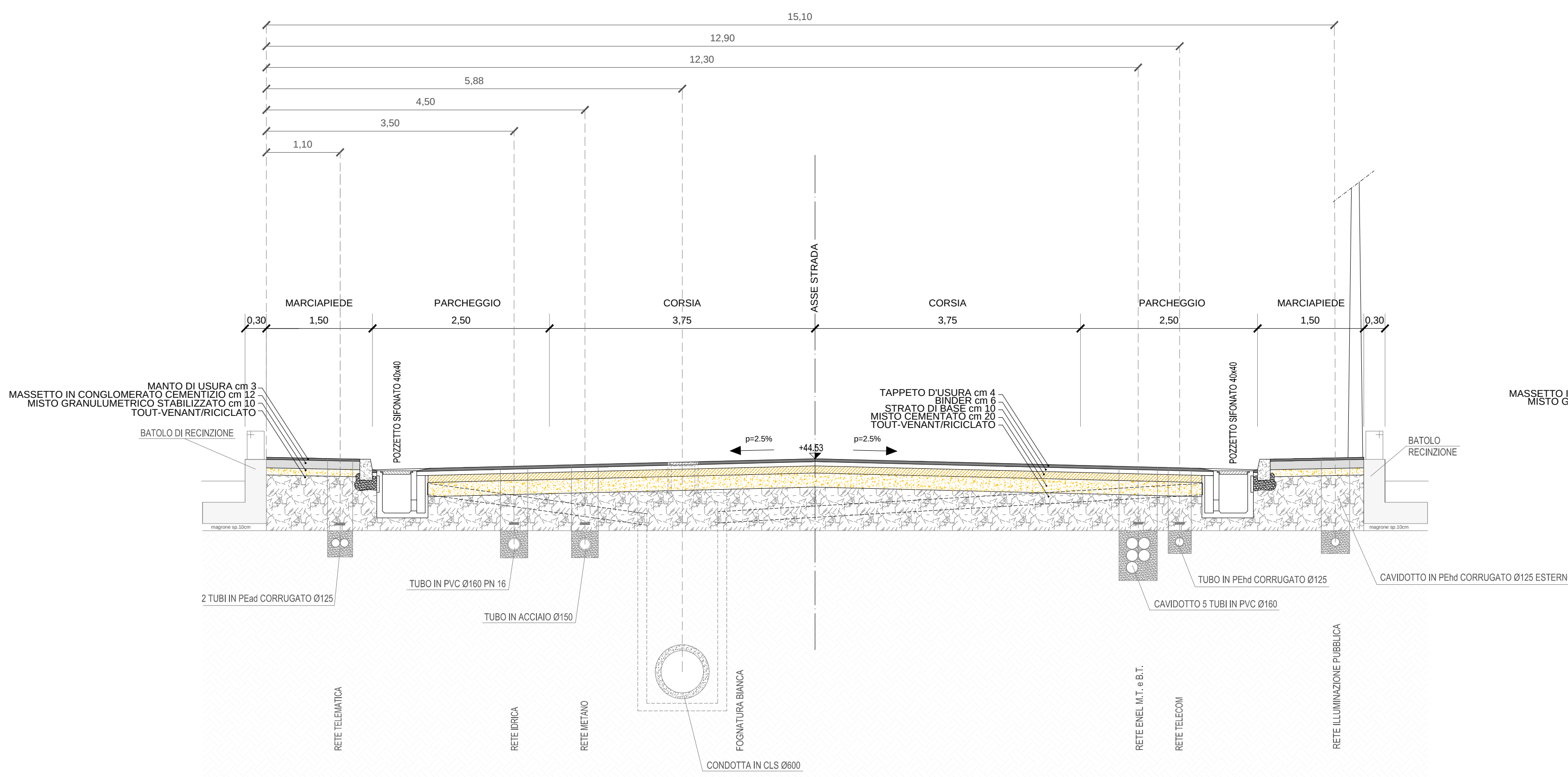
SEZIONE TIPO A-A SCALA 1:50
